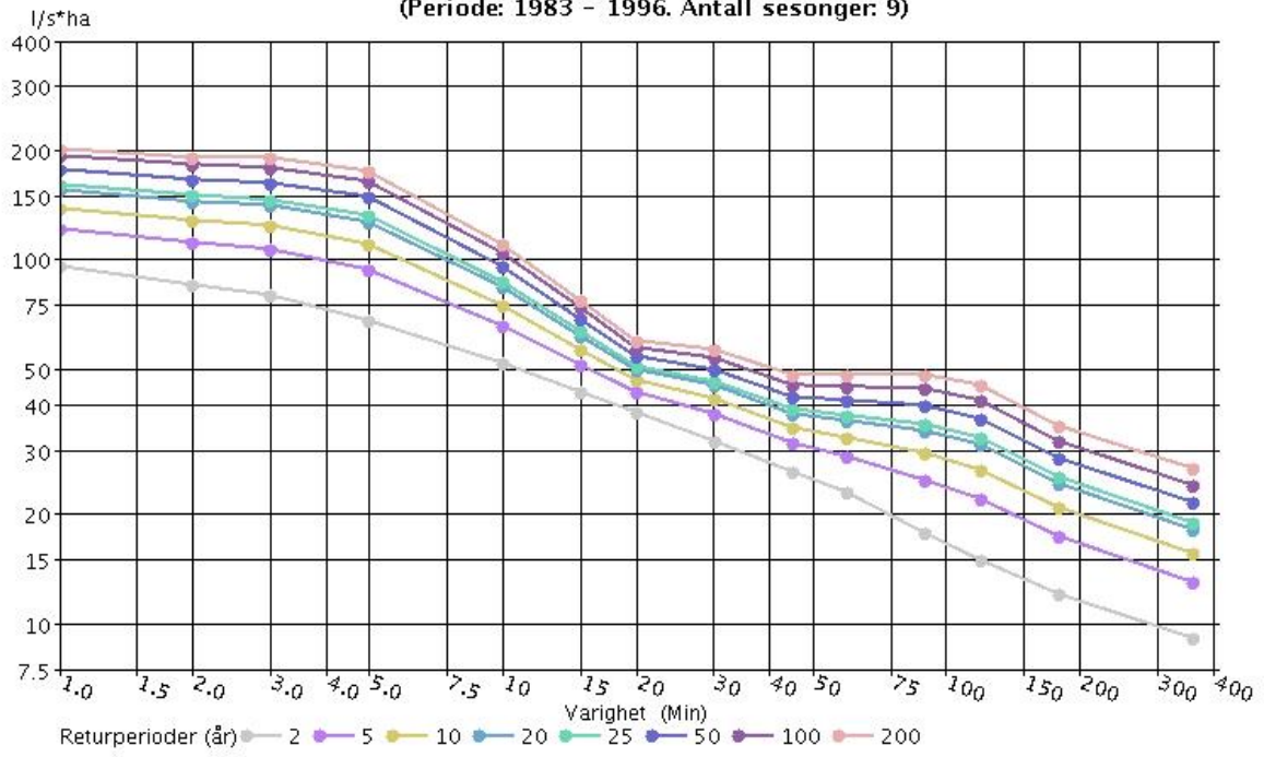
IVF-kurve for 84710 NARVIK - STASJONSVN. (Periode: 1983 - 1996. Antall sesonger: 9)
